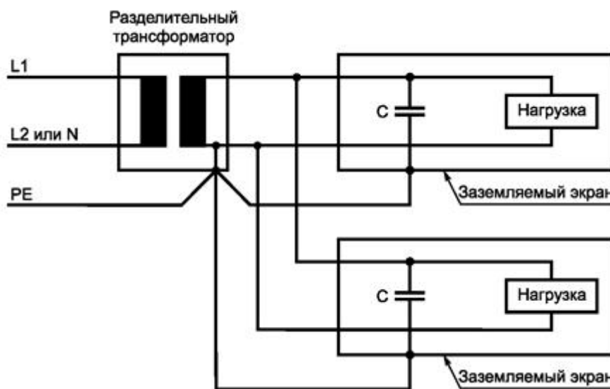
Примечание - Присоединенное оборудование получает питание от основного Рисунок А.1 - Границы между электроустановкой и оборудованием обработки информации
