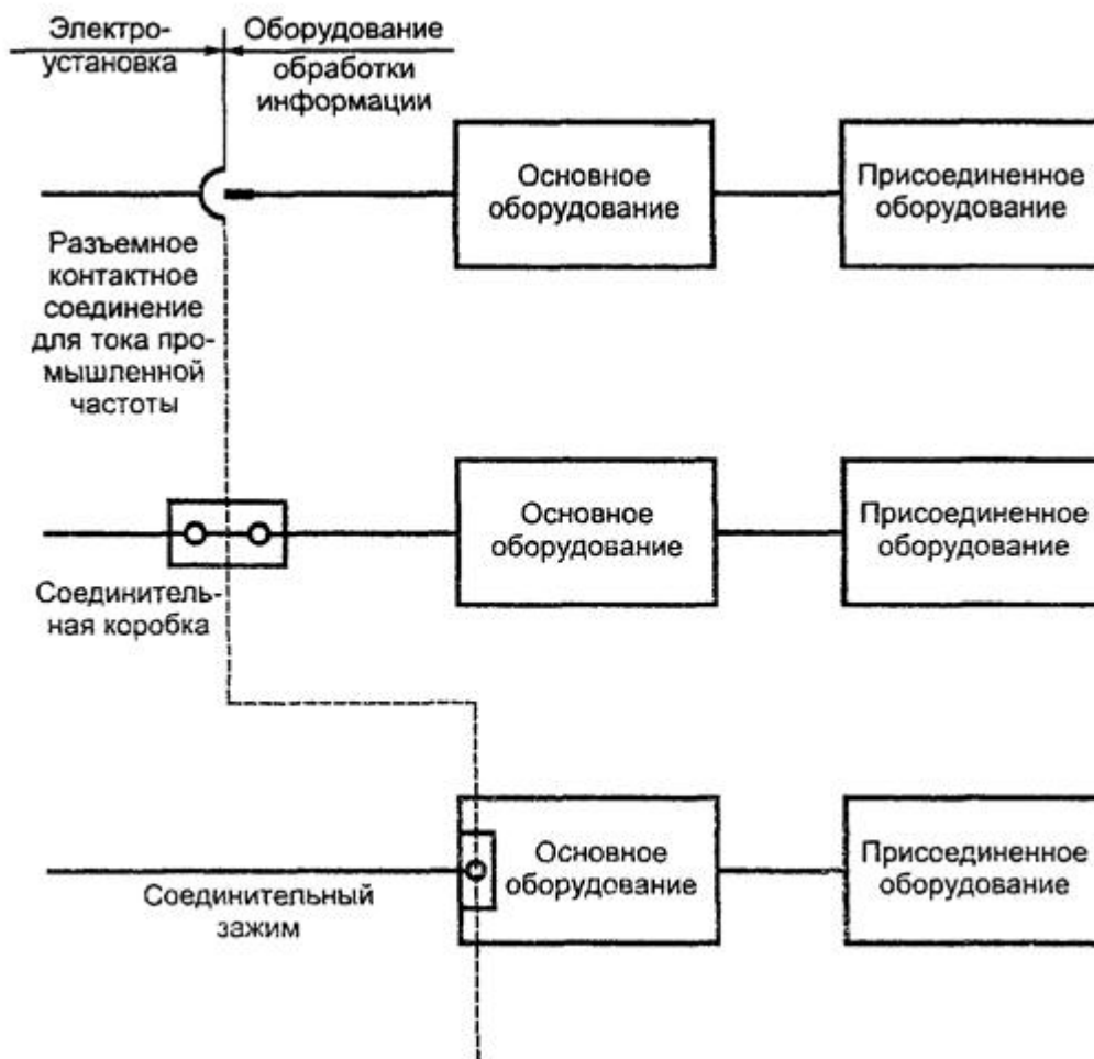
Примечание - Присоединенное оборудование получает питание от основного Рисунок А.1 - Границы между электроустановкой и оборудованием обработки информации
