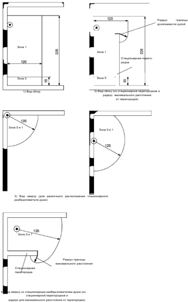
Рисунок 701.2 – Размеры зоны 0 и 1 в помещениях, содержащих души без пола
