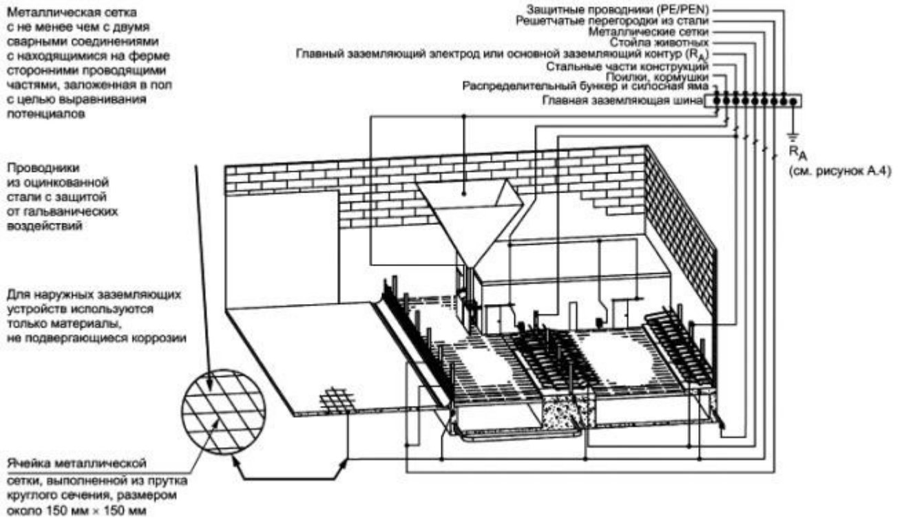
Рисунок А1 - Пример уравнивания потенциалов в коровнике
