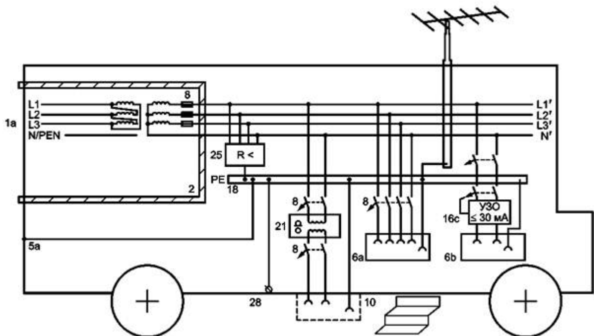
Рисунок 717.7 - Пример соединения со стационарной электрической установкой с любым типом системы заземления, с использованием IT-системы заземления без автоматического отключения после первого замыкания на землю
