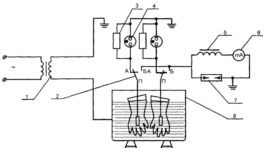
Рис. 2.3. Принципиальная схема испытания диэлектрических перчаток, бот и галош:
