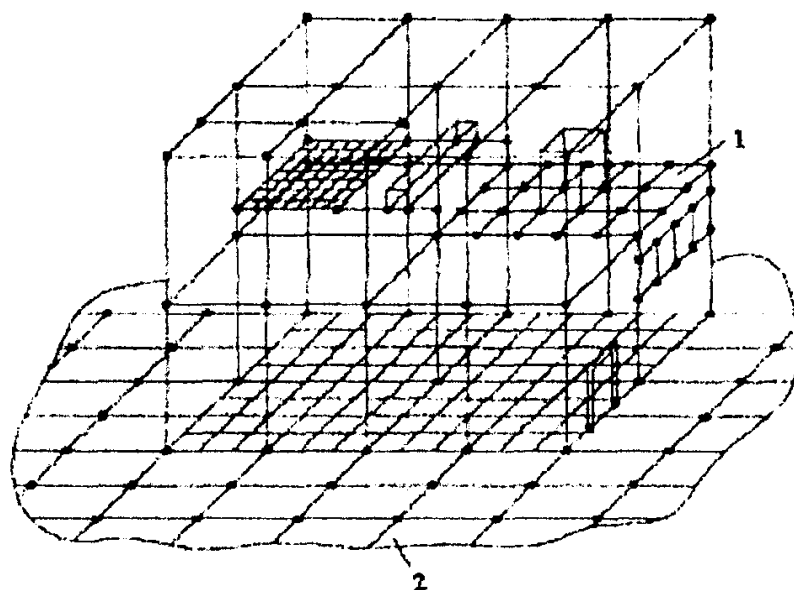
1 - сеть соединений; 2 - заземлитель
